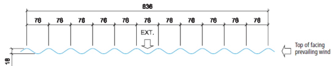
Profil sinus 18/76
