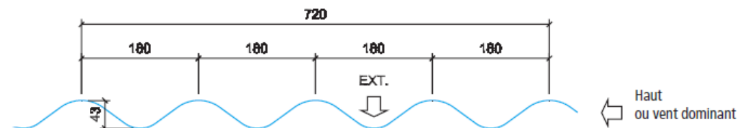
Profil sinus 43/180
